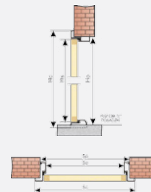
Linia Basic (ościeżnica metalowa-półwłkowa Basic)
